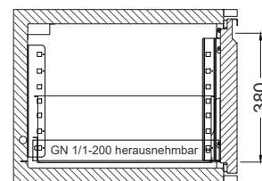
1 Zug mit herausnehmbarem Ladeneinsatz
