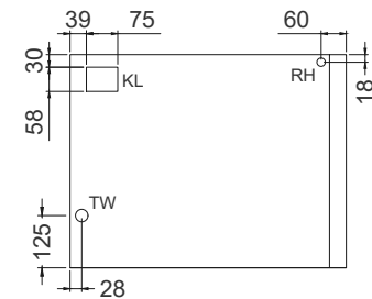
DETAIL LEITUNGSAusGÄNGE in der Seitenwand zum Maschinen-/Installationsfach TW = Tauwasser KL = Kälteleitungen RH = Rahmenheizung ⚡ Elektro- und Steueranschluss
