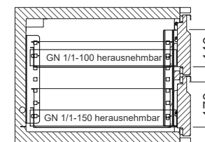
2 Züge 1/2-1/2 mit herausnehmbaren Ladeneinsätzen
