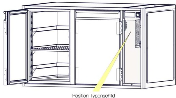
Abbildung 2: Position Typenschild
