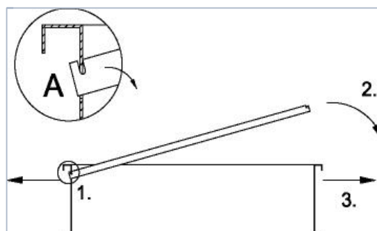
Abbildung 11: Flaschentrennstäbe einsetzen
