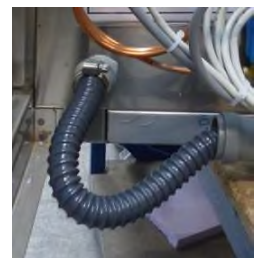
Abbildung 6: Geruchsverschluss
