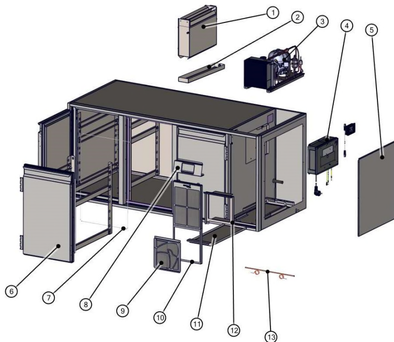
Abbildung 23: Teileübersicht
