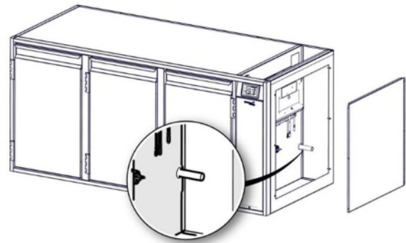
Abbildung 5: Tauwasseranschluss
