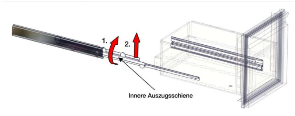
Abbildung 20: Auszugsschiene drehen.
