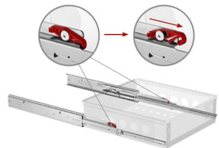
Abbildung 17: Sicherungshebel
