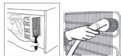
Abbildung 14: Kondensator reinigen
