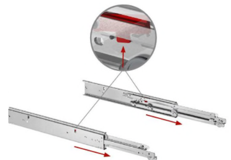
Abbildung 19: Hintere Sicherungslasche
